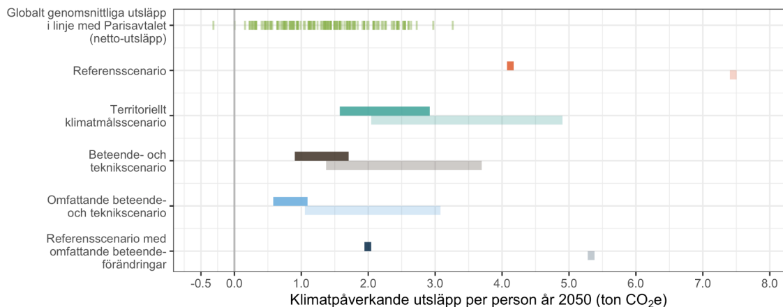
Figur 4 Överst globala genomsnittliga utsläpp i linje med Parisavtalet förutsatt globalt jämlika utsläpp per person. Därefter svenska konsumtionsbaserade utsläpp för de fem scenarierna, först från de analyserade konsumtionsområdena persontransporter, livsmedel samt byggande och boende, och därefter för alla konsumtionsområden (ljusare färg). Högre nivå i spannen: omvärlden utvecklas i linje med nuvarande trender och teknik. Lägre nivå i spannen: en global klimatomställning i linje med Parisavtalet
