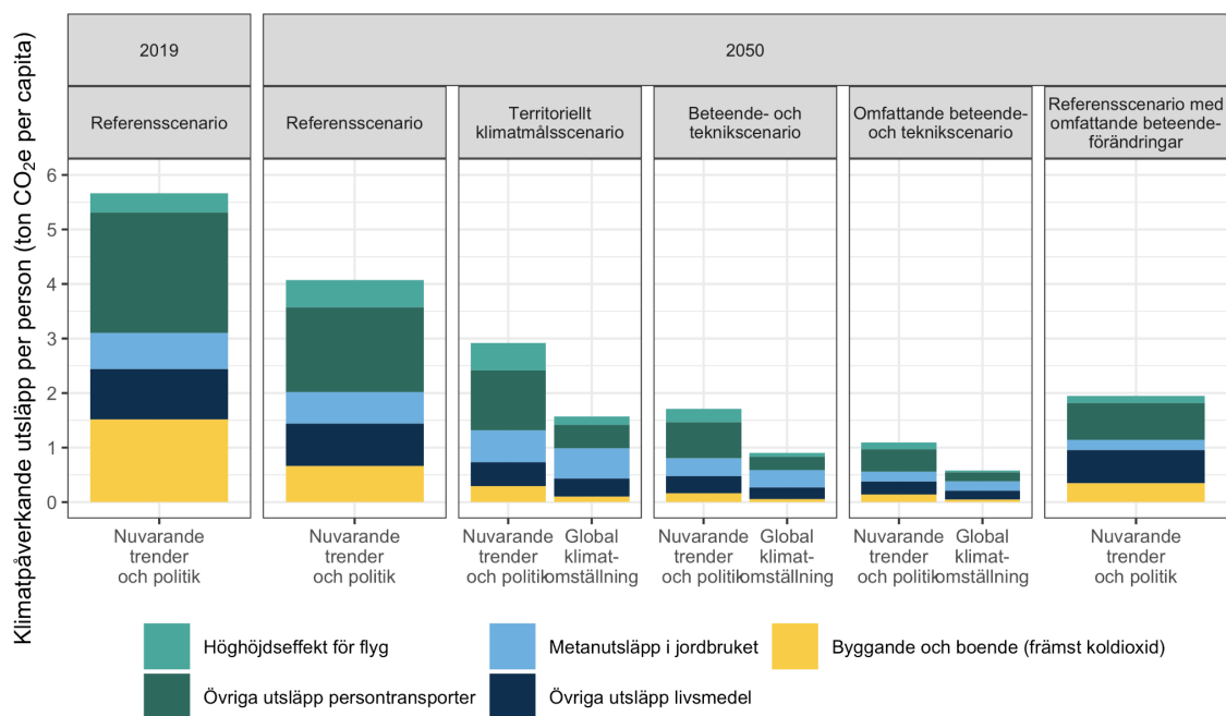
Figur 3 Klimatpåverkande utsläpp per person för respektive scenario år 2050 jämfört med basåret 2019 och fördelat på höghöjdseffekt för flyg, metanutsläpp i jordbruket och övriga utsläpp (främst koldioxid). Metanutsläpp i jordbruket och höghöjdseffekten för flyg bedöms vara de huvudsakliga bidragen till utsläpp av kortlivade växthusgaser för de analyserade konsumtionsområdena.
