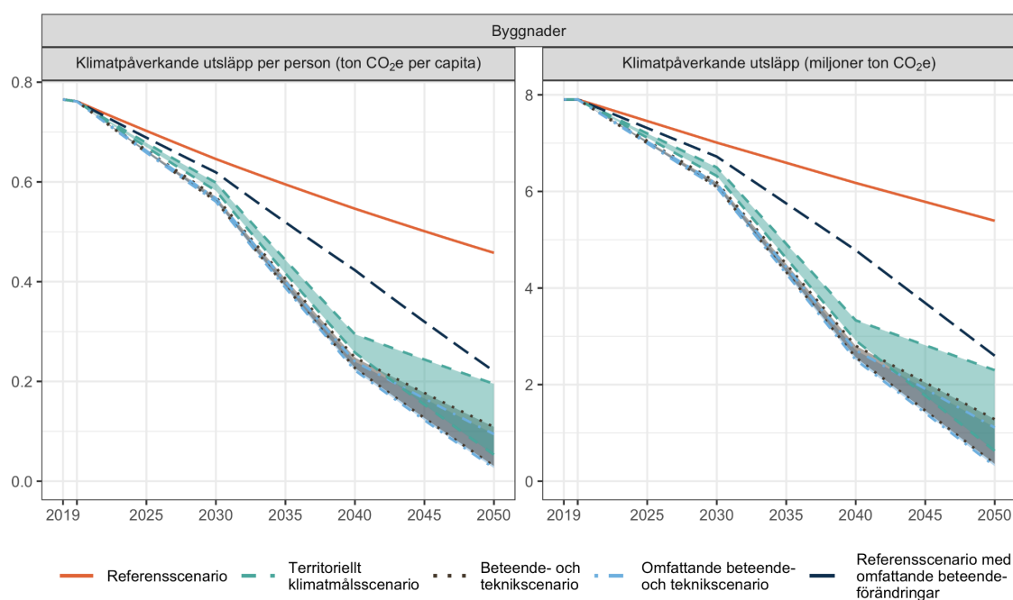
Figur 20 Scenarier för framtida konsumtionsbaserade, klimatpåverkande utsläpp för konstruktion av byggnader i Sverige.
